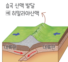
(나) 수렴형(충돌형) 경계 천발~중발 지진 발생
