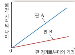
판 경계에서 멀어질수록 해양 지각의 나이가 증가한다. ⇒ 해령에서 지각이 생성된다.
