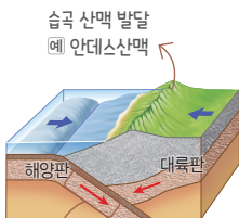
(가) 수렴형(섭입형) 경계 천발~심발 지진 발생
