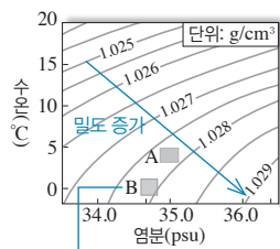
(나) 밀도: A < B → A는 북대서양 심층수(㉠), B는 남극 저층수(㉡)
