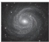
(가) 세이퍼트 은하
