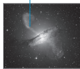
(다) 전파 은하
