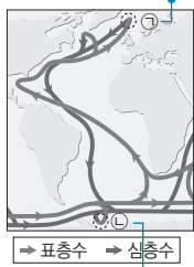
(가) 웨일해, 남극 저층수 형성 밀도: 북대서양 심층수 < 남극 저층수
