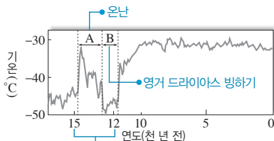
기온: A > B → 수온: A > B → 해수의 평균 밀도: A < B
