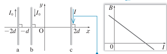
(가) O에서 c에 흐르는 전류에 의한 자기장이 ⊗일 때의 전류 방향이다.
