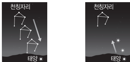
● 별자리 이동(태양 기준) → 이동 방향: 동 → 서 (계절에 따른 별자리 변화) ● 태양의 이동(별자리 기준) → 이동 방향: 서 → 동 (태양의 연주 운동)
