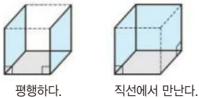
평행하다. 직선에서 만난다.
