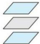
평행하다. 한 점에서 만난다. 꼬인 위치에 있다.
