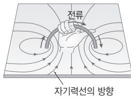
자기력선의 방향
